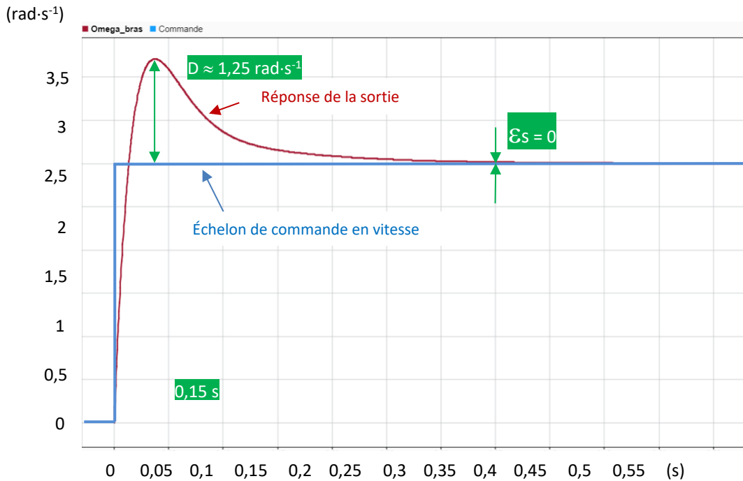
Figure 23 : réponse à un échelon de vitesse de la structure multi-physique du bras 1 en boucle fermée.
