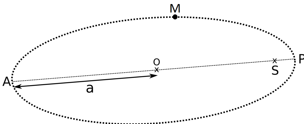
figure 7. Orbite elliptique de la sonde PSP en 2025
