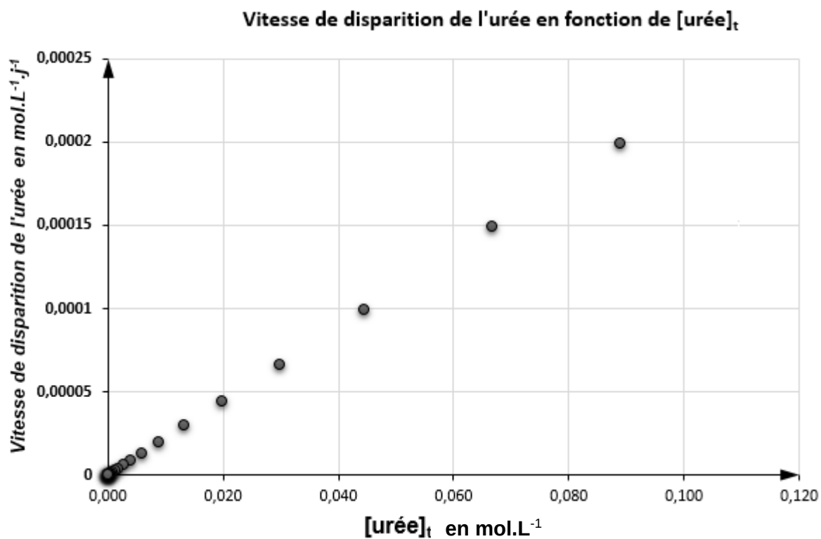
figure 3 : évolution de la vitesse volumique de disparition de l'urée en fonction de la concentration en urée, [urée]_t
