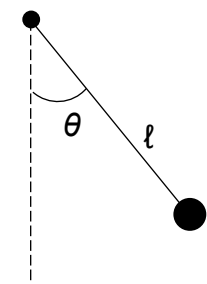
Schéma d'un pendule simple
