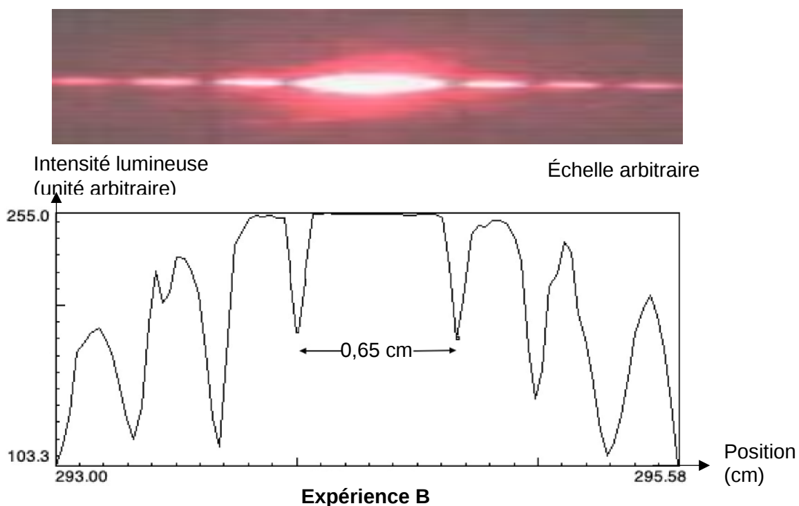
Figure 2. Photographies des figures de diffraction obtenues et distribution de l'intensité lumineuse pour deux fils calibrés de diamètres différents.
