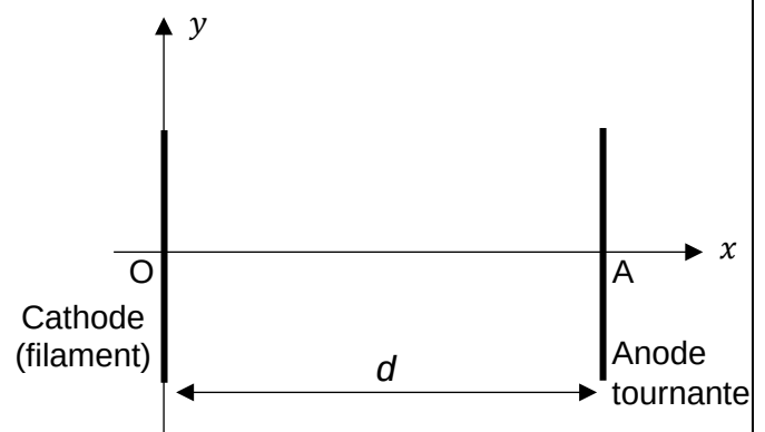
Figure 2 - Schéma simplifié
