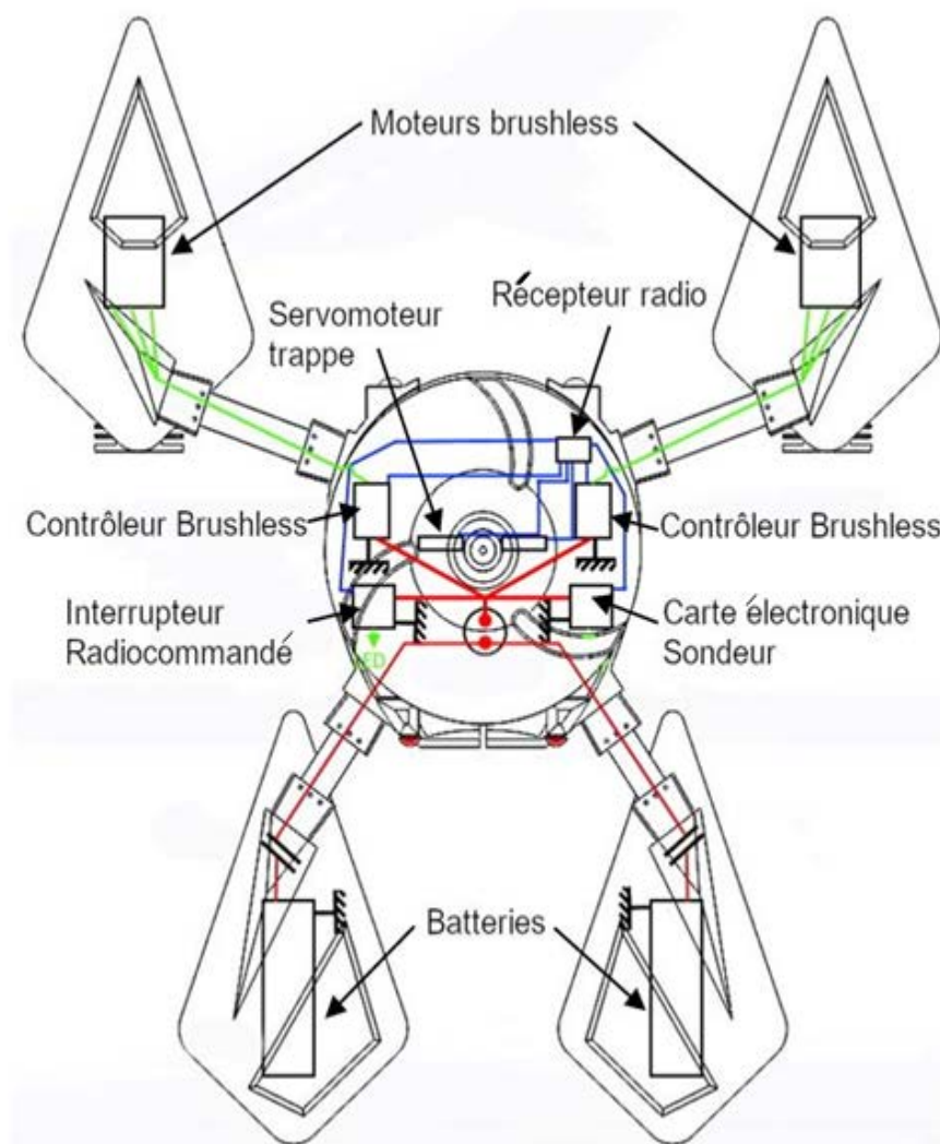
figure 19 : représentation simplifiée des éléments électriques
