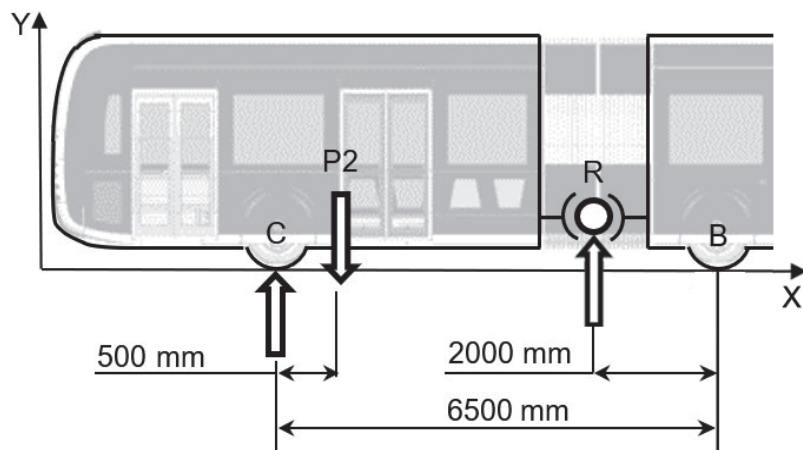
Figure 10 : schéma statique de répartition des charges sur l'arrière
