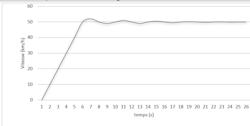
Figure 13 : courbe de régulation de vitesse pour une consigne de 50 km·h -1
