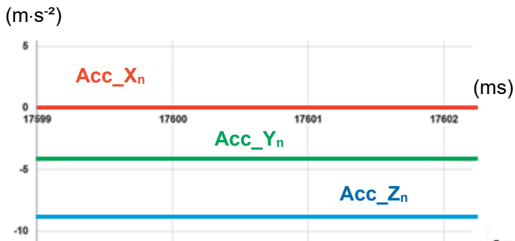
Figure 8 : graphe et données accélérométriques (en \text{m}\cdot\text{s}^{-2} ) en fonction du temps (en ms) pour la position stable de la sonde fictive.
