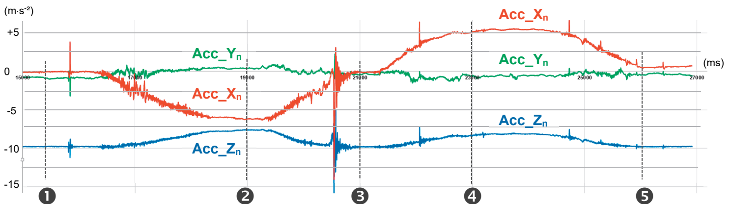
Figure 7 : données accélérométriques (en m.s^{-2} ) en fonction du temps (en ms)
