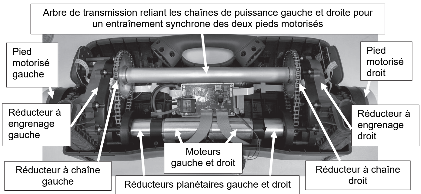
Figure 6 : chaînes de puissance côtés gauche et droit à l'intérieur de l'assise
