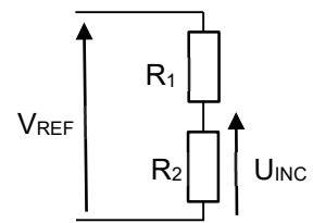
Figure 21 : production d'une tension image de l'angle d'inclinaison.
