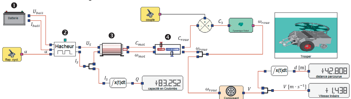
Figure 6 : modélisation multiphysique de la chaîne de puissance
