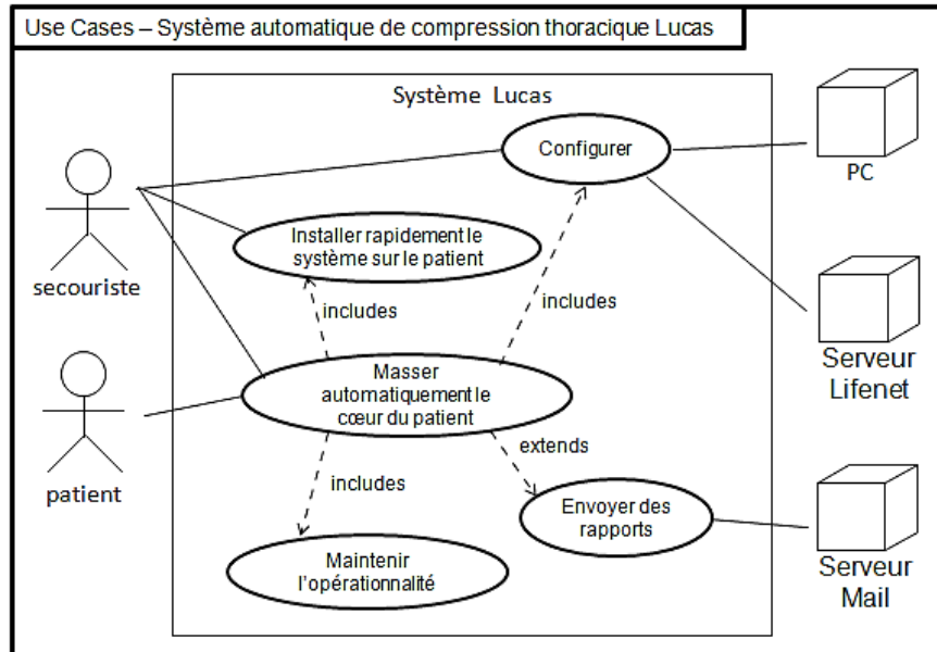
figure 4 - Diagramme des cas d'utilisation
