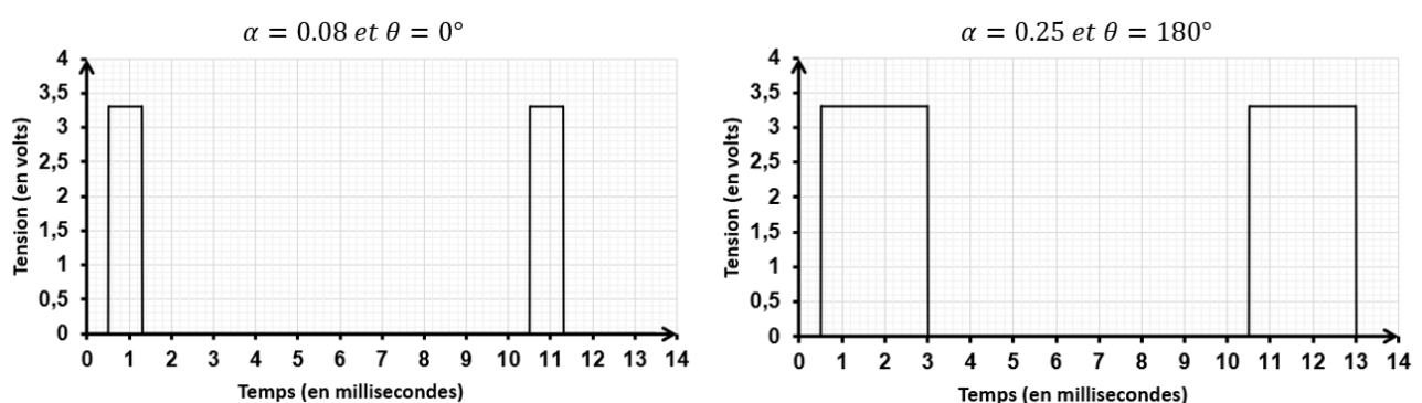
Figure 22 : signal de commande MLI du servomoteur
