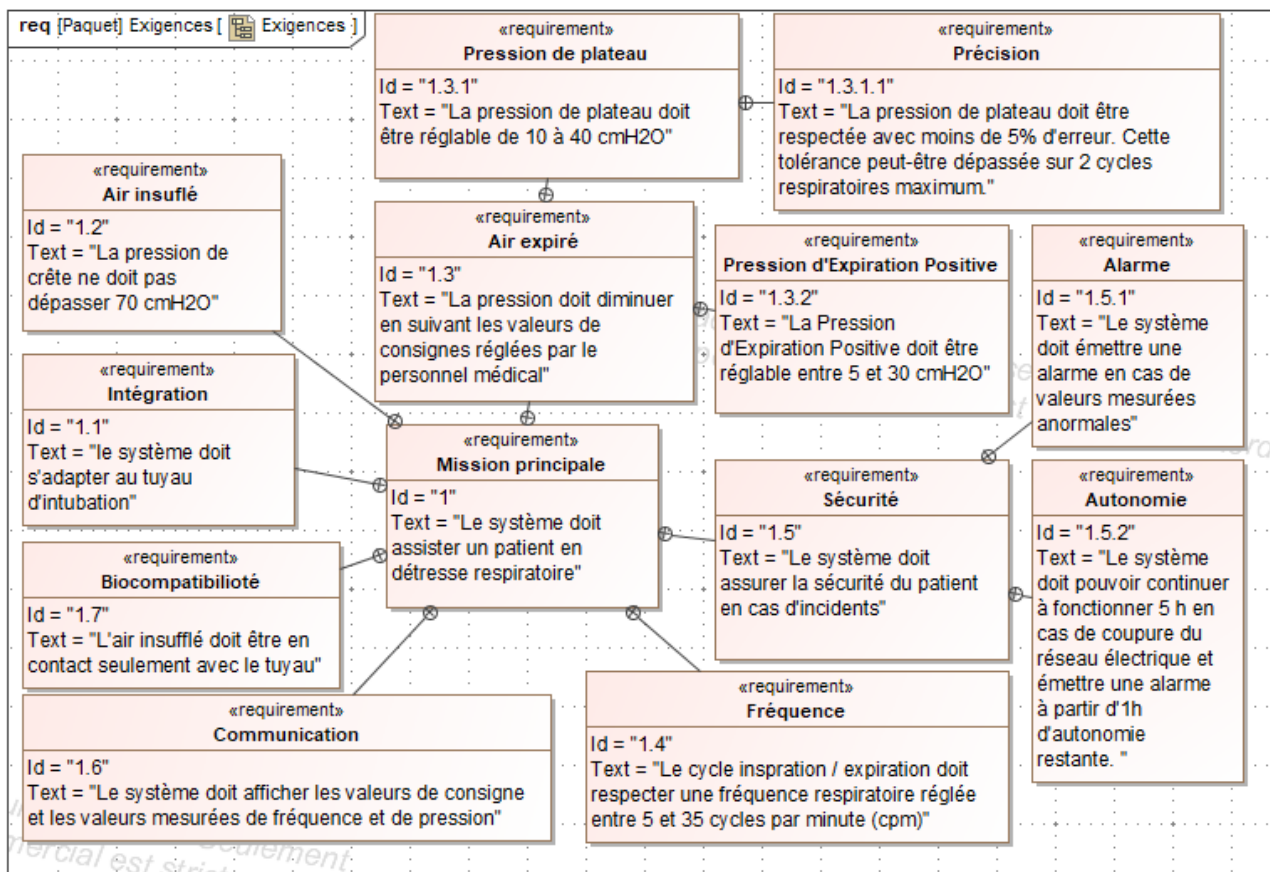
Figure 5 : diagramme partiel d'exigences du MakAir
