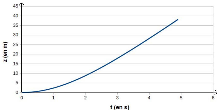
Figure 2. Évolution de la position du centre de masse du grêlon en fonction du temps
