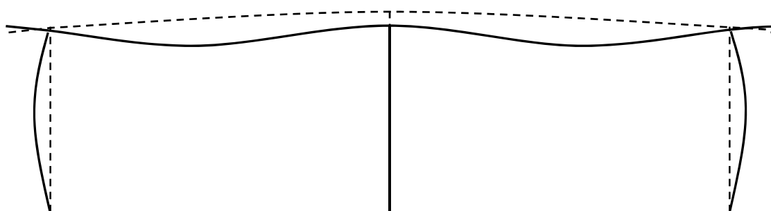
Déformée portique BLC
