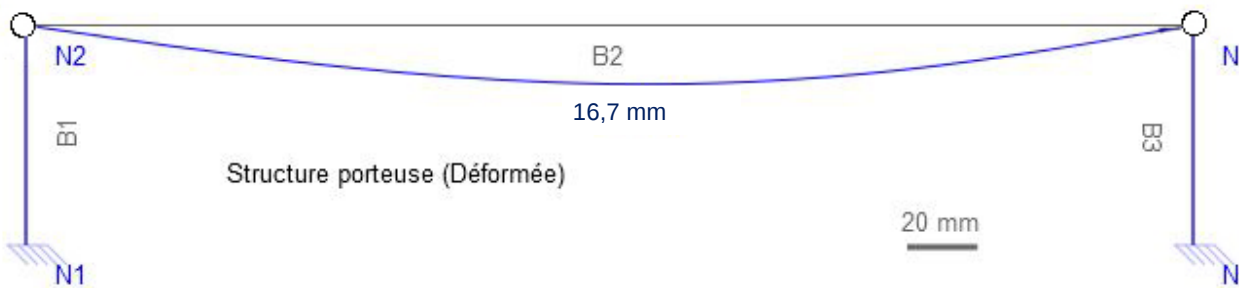
Déformée de la structure porteuse modèle n°1
