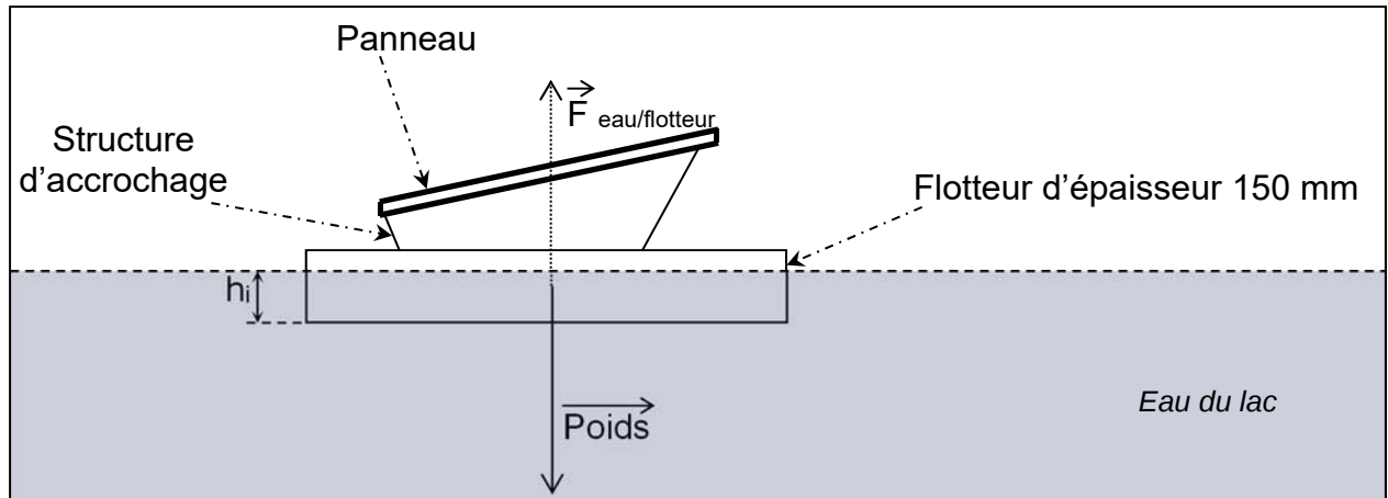
Figure 6 : Schéma mécanique de flottaison
