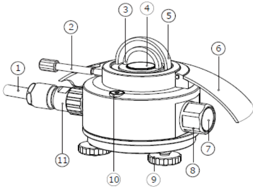
(1) câble, (2) fixation de l'écran de protection solaire, (3) Dôme intérieur, (4) capteur thermique avec revêtement noir, (5) dôme extérieur, (6) écran de protection solaire, (7) indicateur d'humidité, (8) cartouche remplie de déshydratant, (9) pieds réglables, (10) niveau à bulle, (11) connecteur
