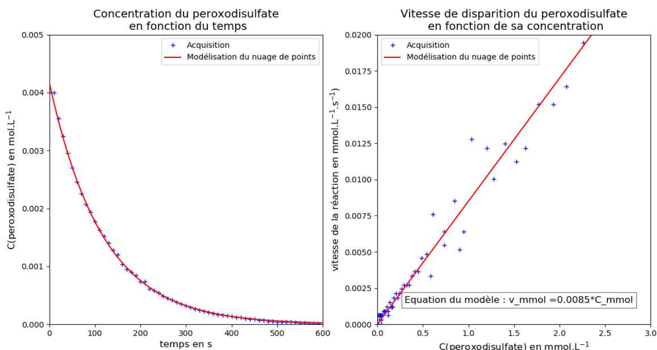
Figure 1 : étude cinétique de l'oxydation des ions iodure par les ions peroxydisulfate
