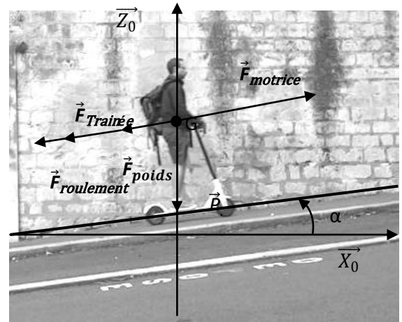
Figure 3: Bilan des actions mécaniques
