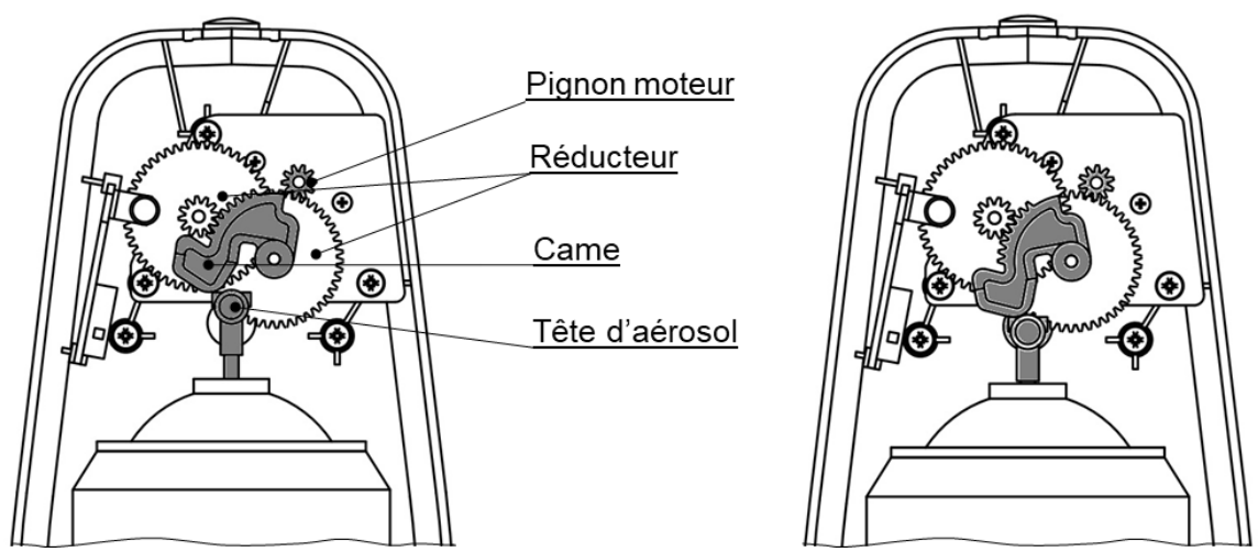
Figure 1.c : positions relâchée et enfoncée de la tête d'aérosol.
