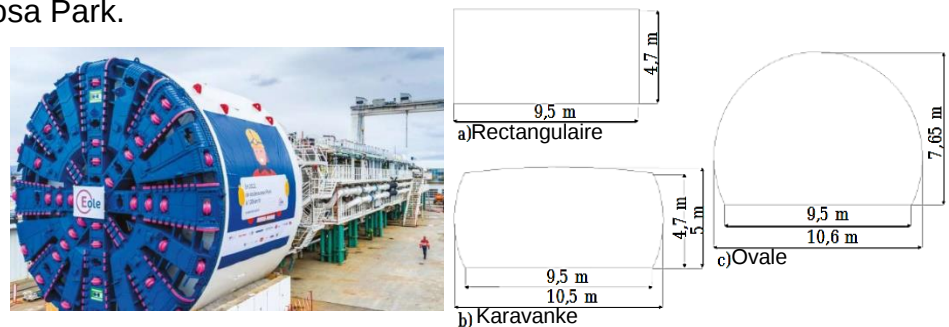
Figure II-1 : Foreuse du tunnelier – Types de tunnel ferroviaire
