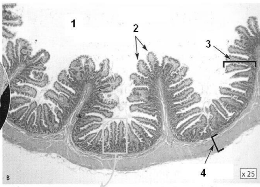
L'intestin grêle vu en coupe (A) et détail de l'intestin grêle en coupe (B).
