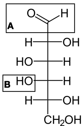
D-Galactose
