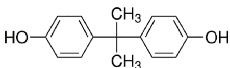
Bisphénol A
