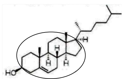
Molécule 3
