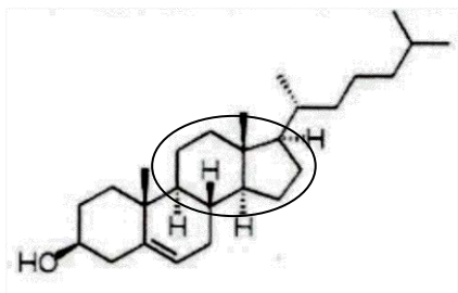
Molécule 1
