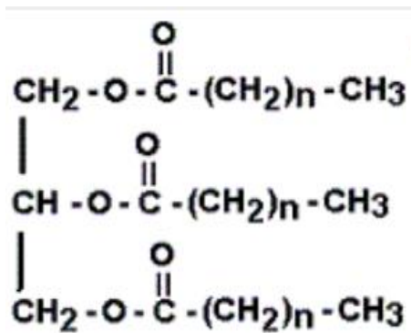
(A) Triglycéride
