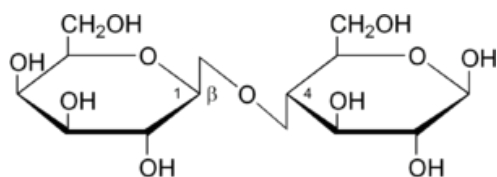
Lactose
