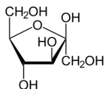
D-Fructose
