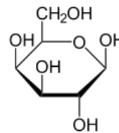
D-Galactose
