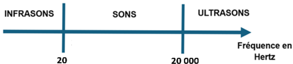
Document n°4 : domaines de fréquences des ondes sonores
