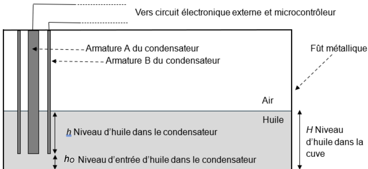
Figure 3. Schéma du dispositif de mesure dans le fût métallique.
