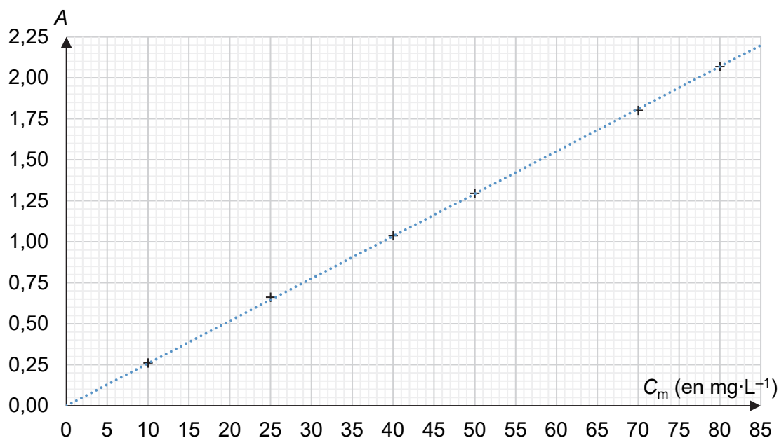
Figure 1. Courbe d'étalonnage de l'acide salicylique dans le collyre à \lambda = 295 \text{ nm}
