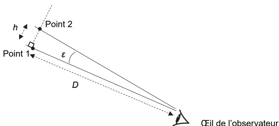
Figure 1. Construction géométrique permettant de déterminer l'angle \varepsilon sous lequel on voit deux points distants de h , observés à une distance D
