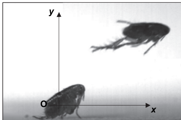
Figure 1. Extrait de la chronophotographie du saut de la puce.
