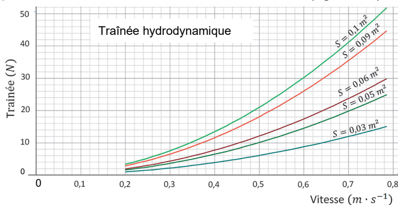
Figure 10 : action mécanique de trainée
