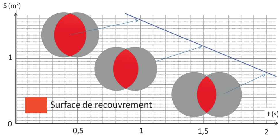
Figure 14 : surface de recouvrement en fonction du temps entre deux mesures à la vitesse de nettoyage d'un nœud
