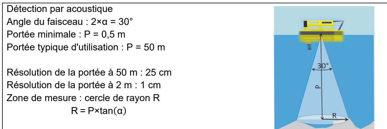
Figure 13 : géométrie de la zone de mesure
