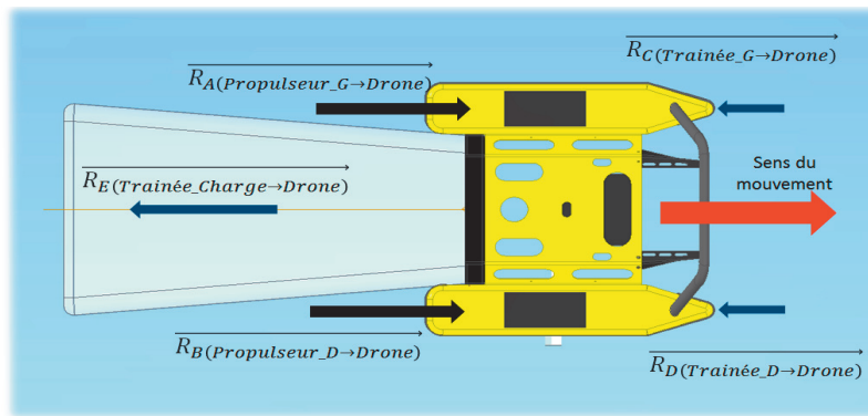
Figure 9 : actions de poussées et de trainées
