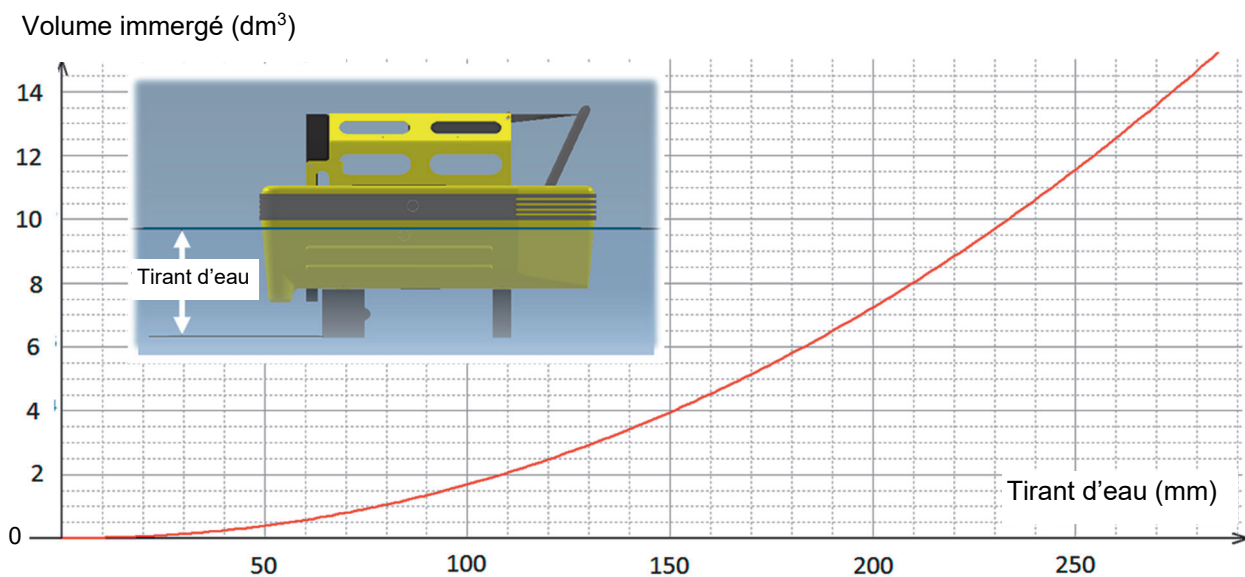
Figure 8 : volume immergé d'un seul flotteur en fonction du tirant d'eau
