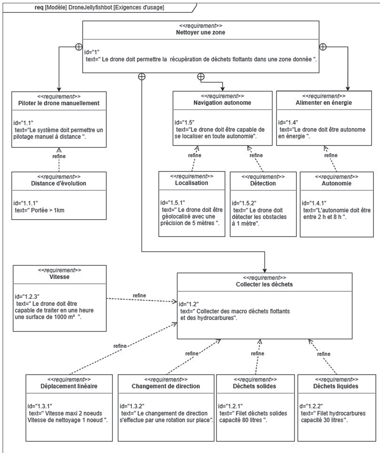
Figure 3 : diagramme des exigences du drone
