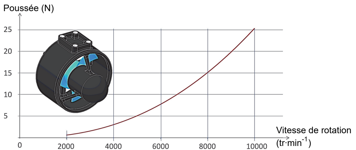
Figure 11 : poussée d'un propulseur
