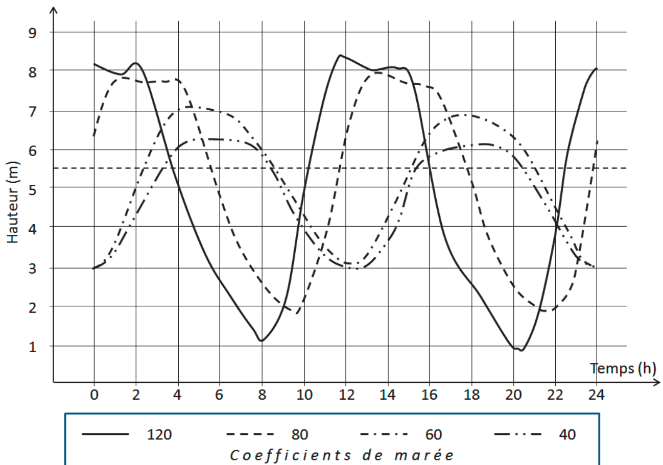
Figure 5 : hauteur d'eau en fonction du temps pour différents coefficients de marée
