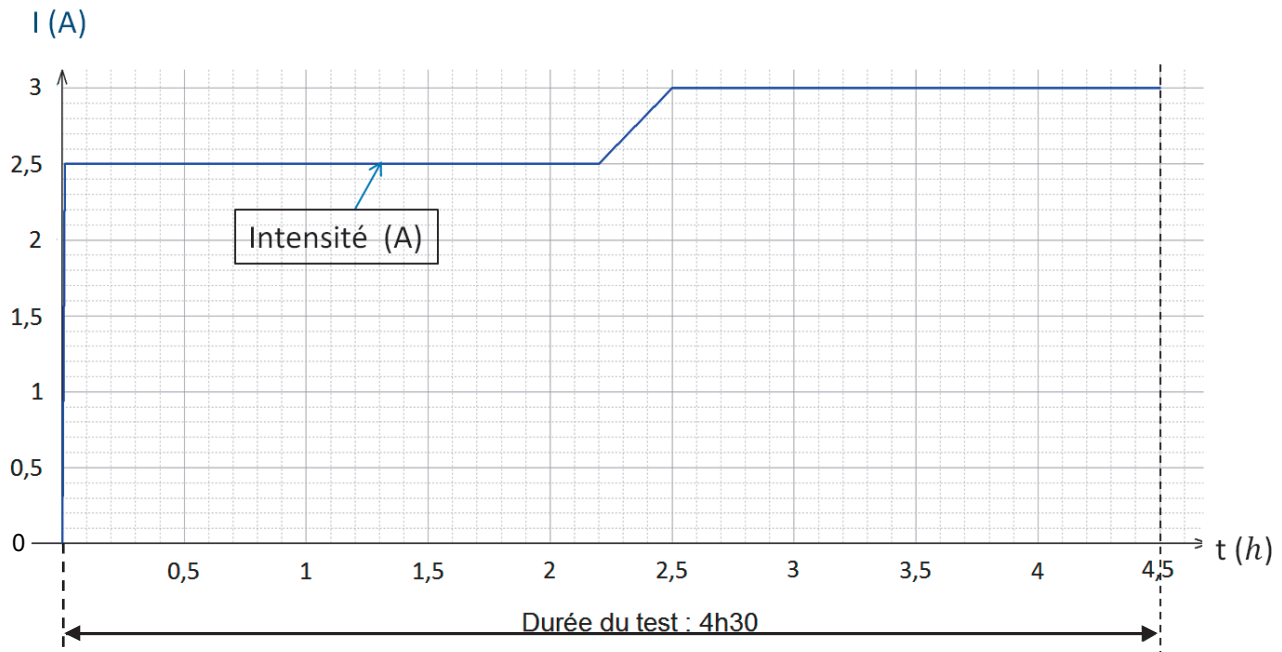
Figure 7 : intensité du courant consommée par le propulseur A
