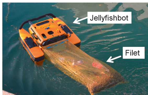
Figure 1 : robot en cours de collecte
