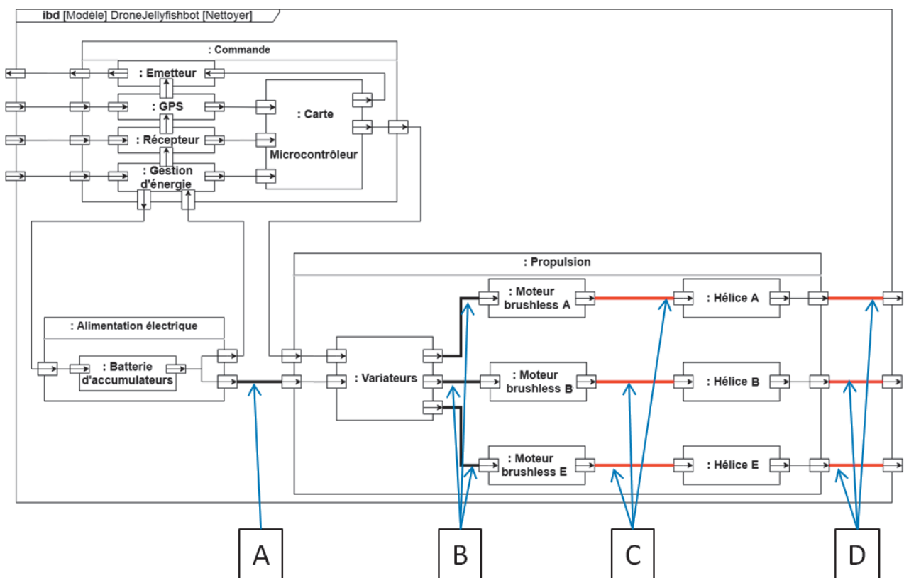
Figure 4 : diagramme de blocs internes
